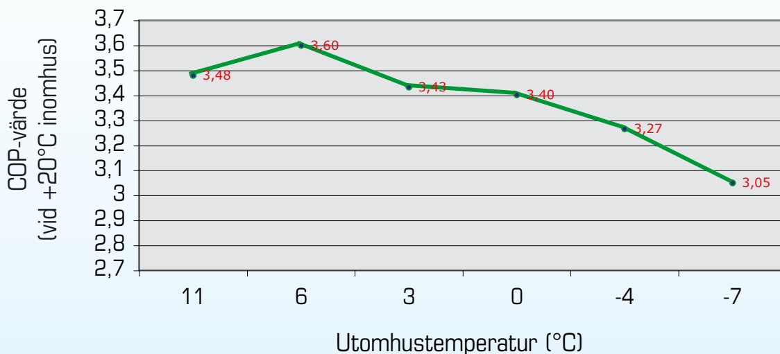
COP-värde vid olika utomhustemperaturer
